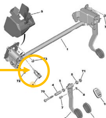
ブレーキライトスイッチ
